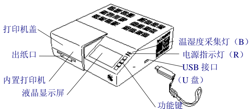
主机外形结构图 (正面图)
